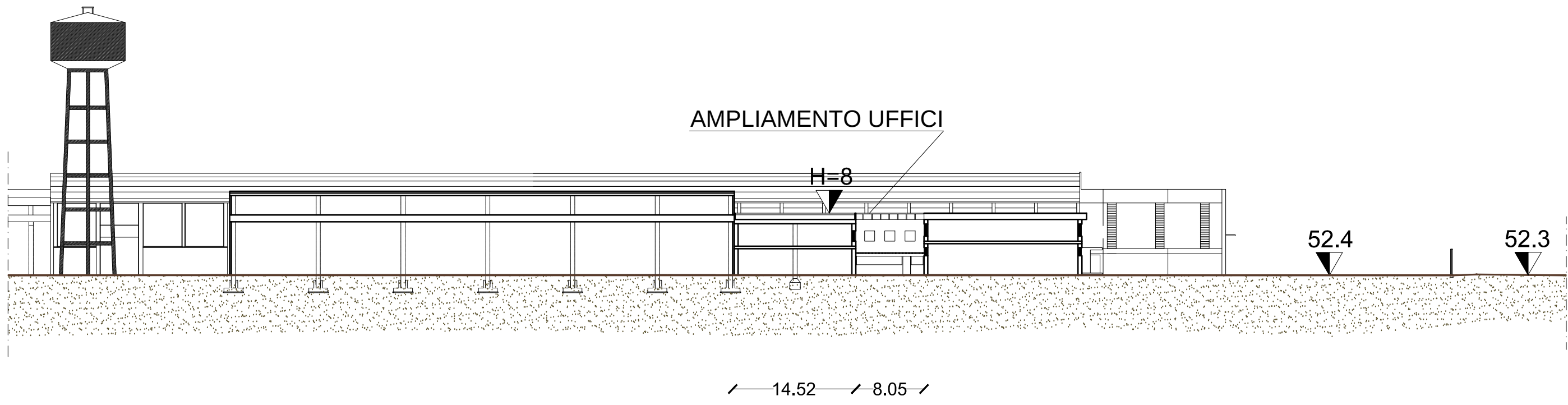
SEZIONE E-E - scala 1:500
