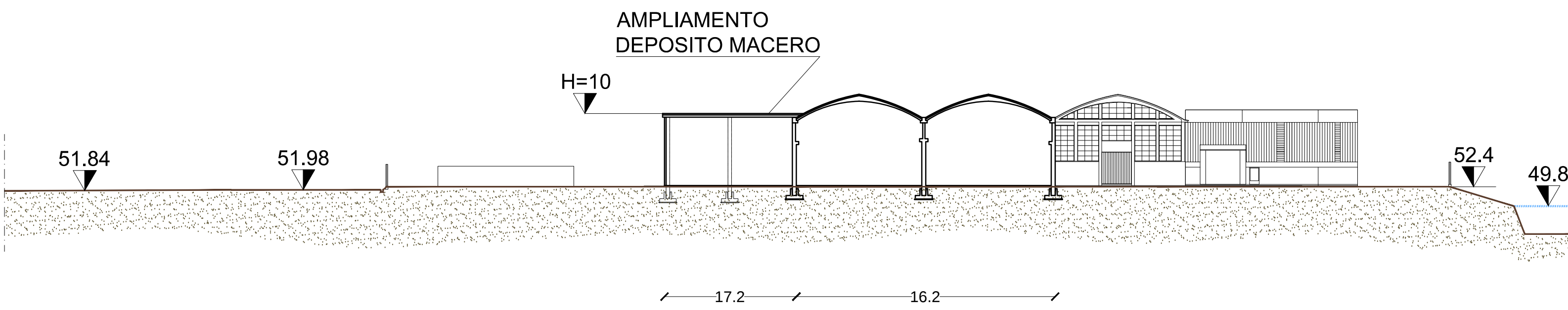
SEZIONE F-F - scala 1:500
