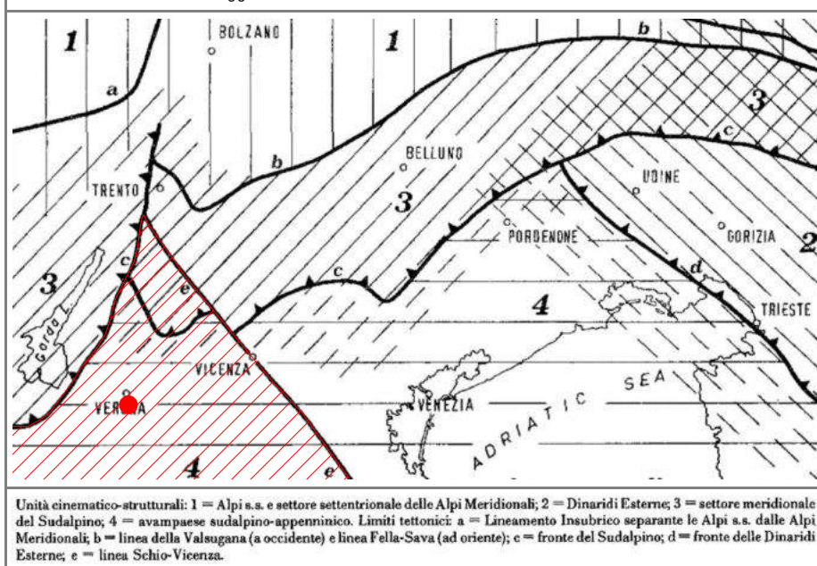
Fig. 18. Carta delle "Unità cinematico - strutturali dell'Italia Nord Orientale" (da Slejko et alii, 1987). In rosso l'ubicazione del sito oggetto di studio.
