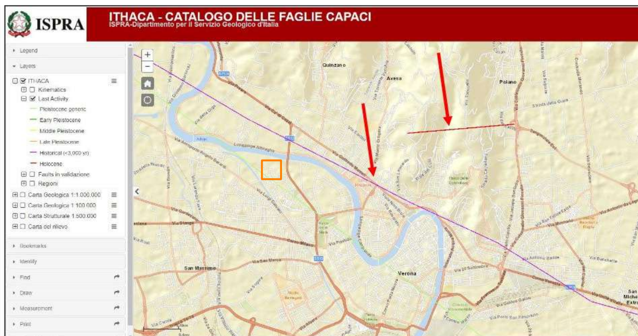
FIG. 39: MICROZONAZIONE SISMICA ESTRATTO DA CATALOGO DELLE FAGLIE CAPACI
