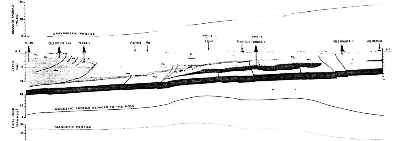
FIG. 20: SCHEMA TETTONICO PIANURA PADANA OCCIDENTALE
