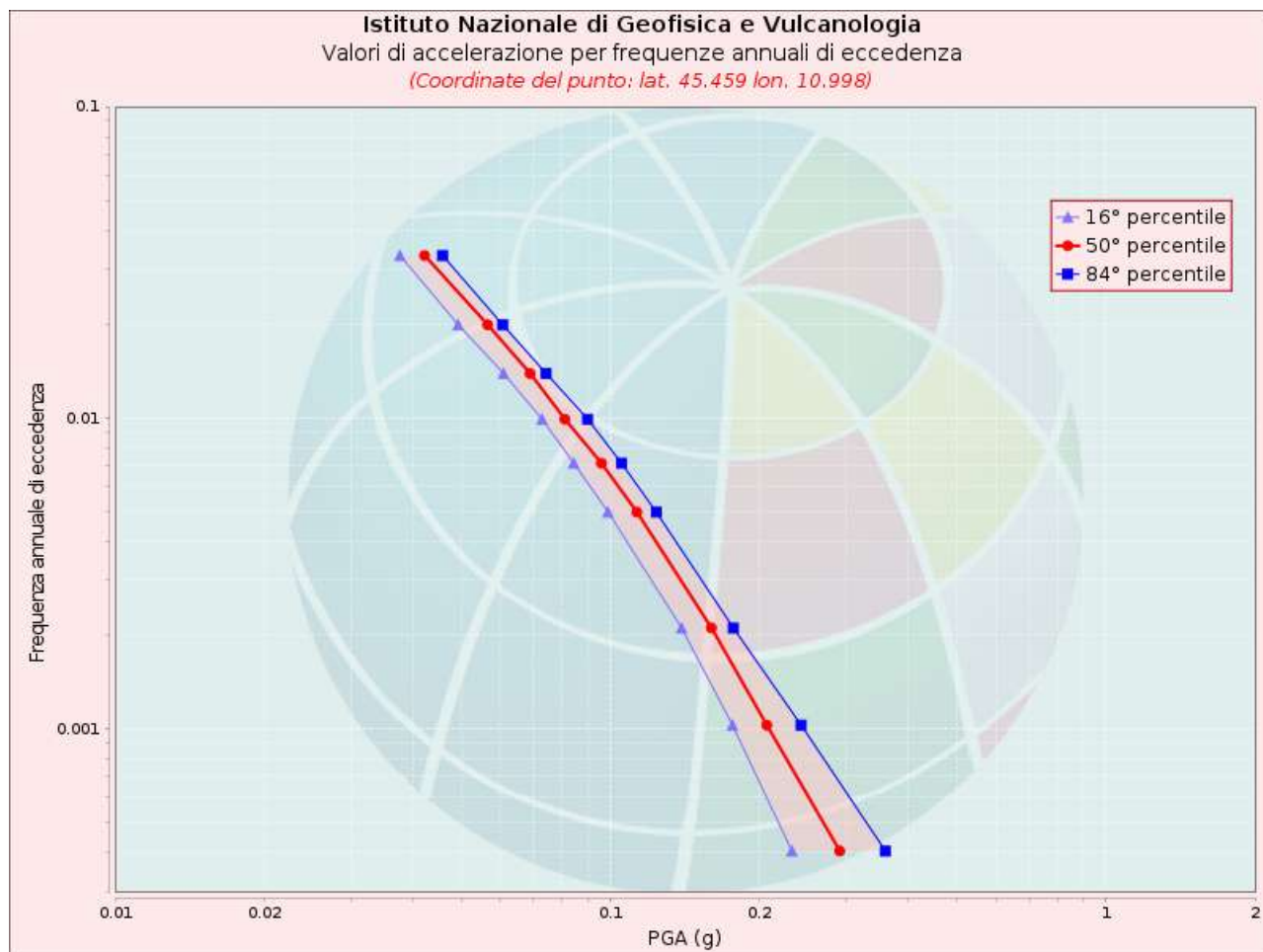
FIG. 23 20 : CURVA DI PERICOLOSITÀ
