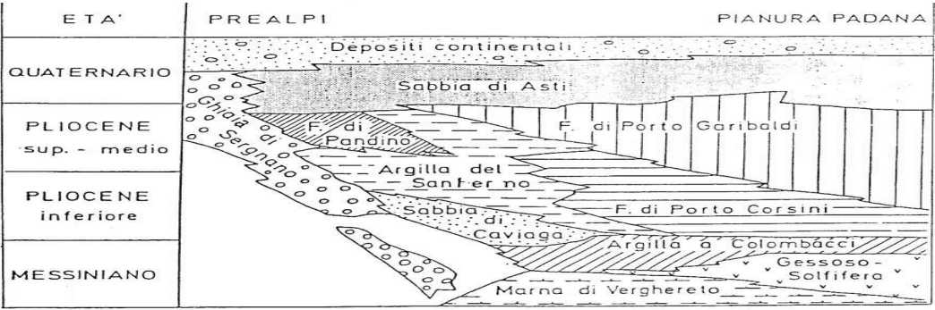
FIG. 19: STRATIGRAFIA SONDAGGIO RODIGO 1 (DA A. CASTELLARIN 1985 – AGIP ).
