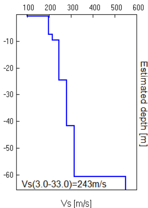
FIG. 29: ANDAMENTO DELLA Vs CON LA PROFONDITÀ
