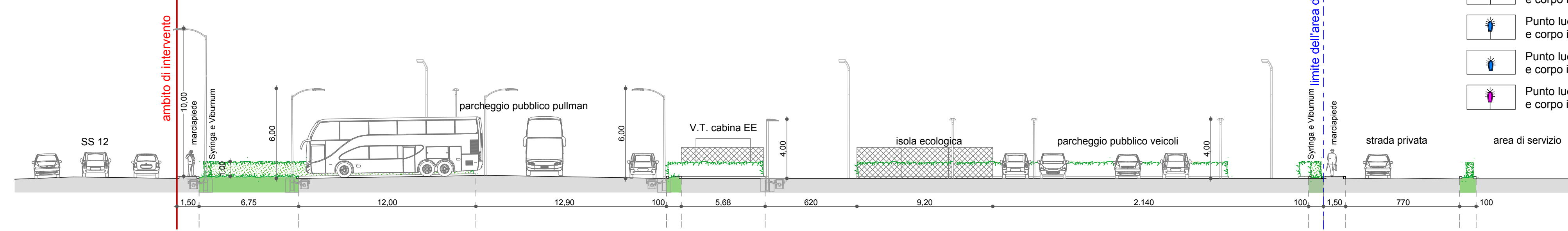
scala 1:200
