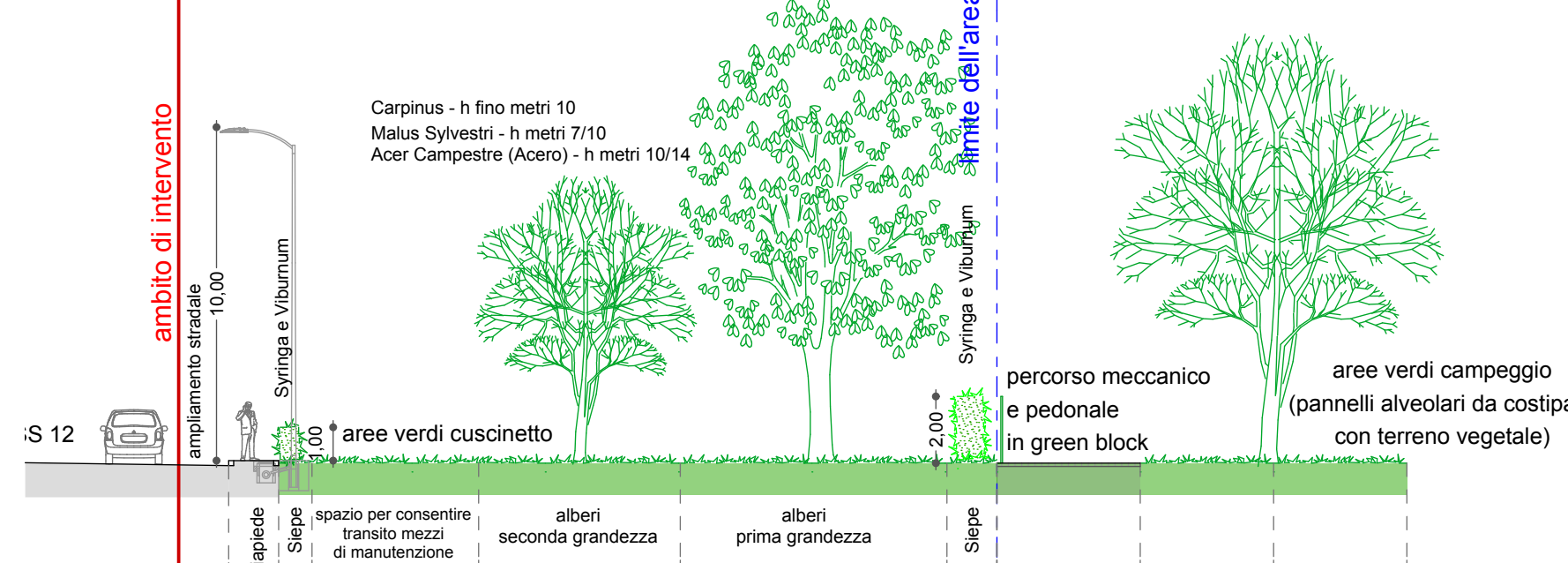
scala 1:200
