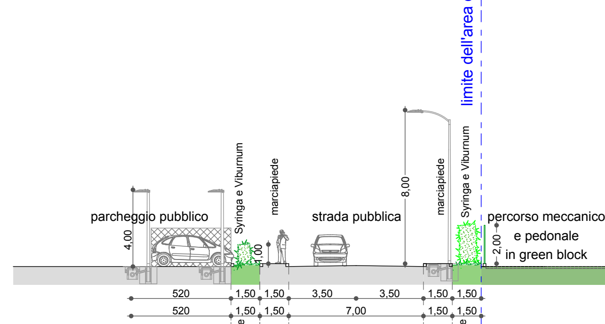
scala 1:200
