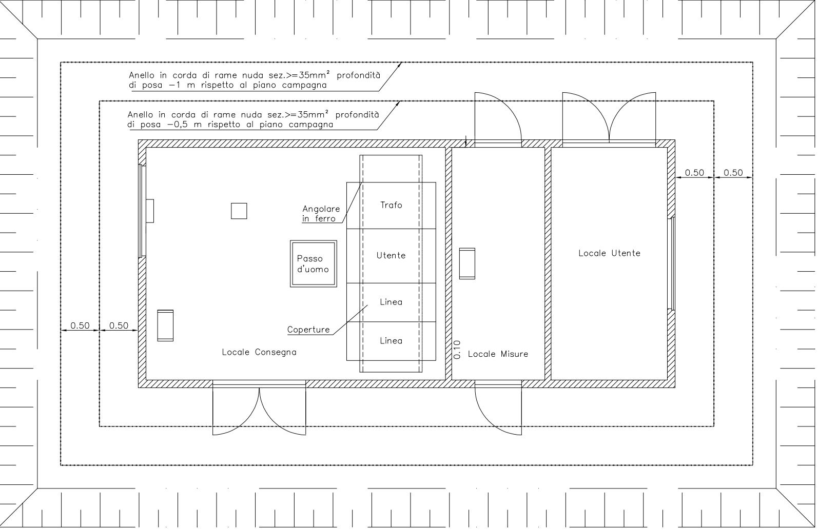
IMPIANTO DI TERRA
