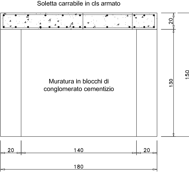
SEZ. B - B
