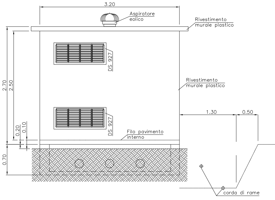
PROSPETTO LATERALE DESTRO
