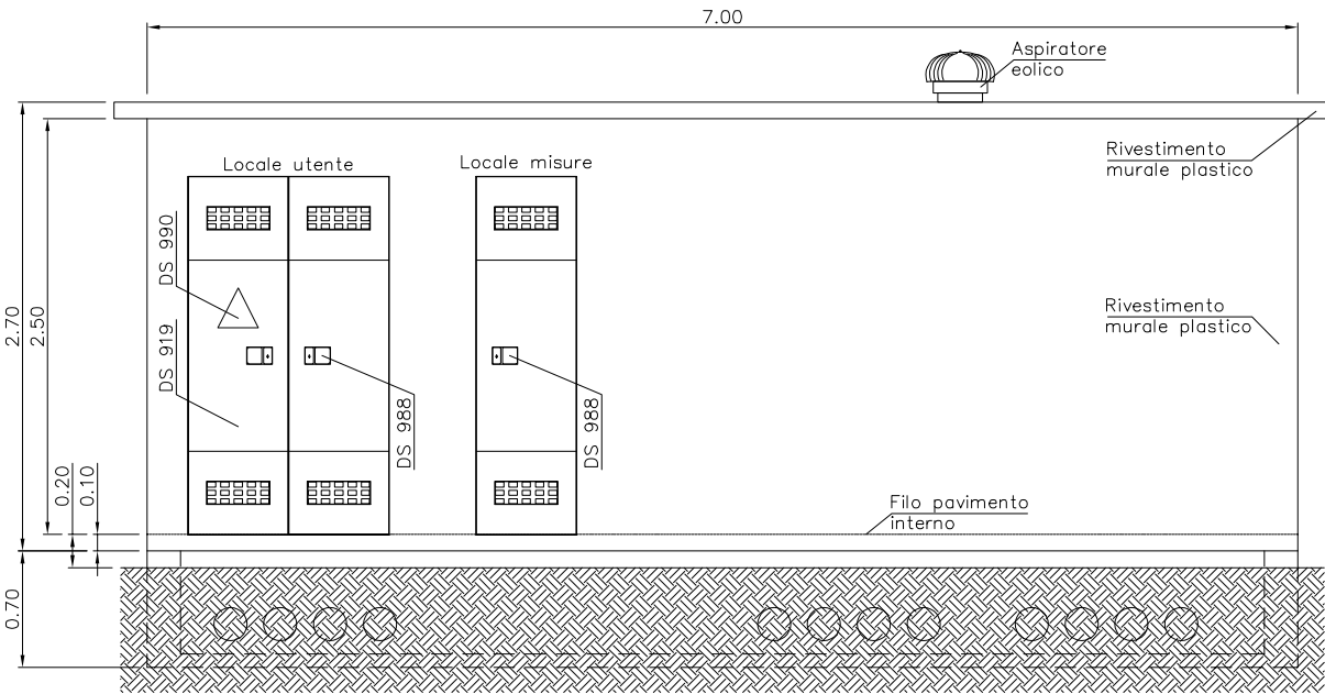
PROSPETTO POSTERIORE
