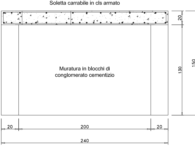
SEZ. A - A
