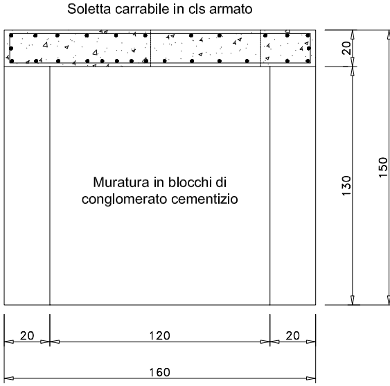
SEZ. B - B
