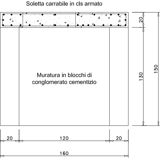
SEZ. A - A
