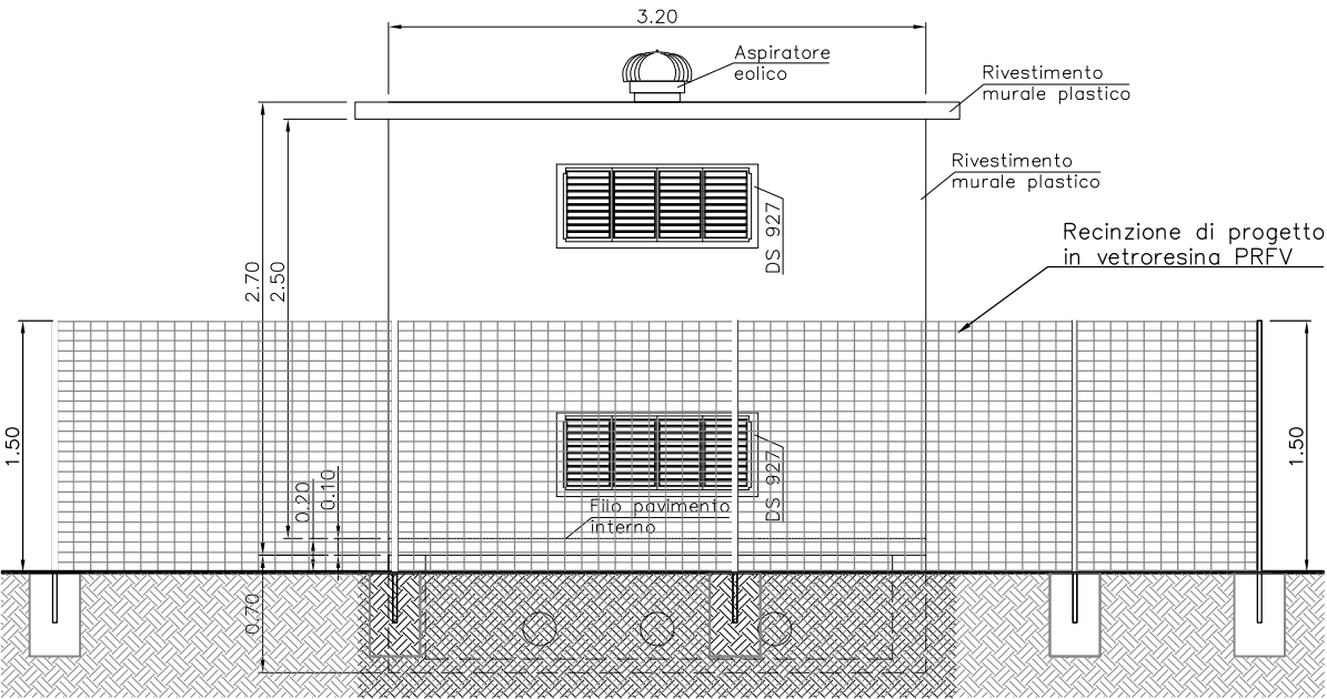
PROSPETTO LATERALE SINISTRO
