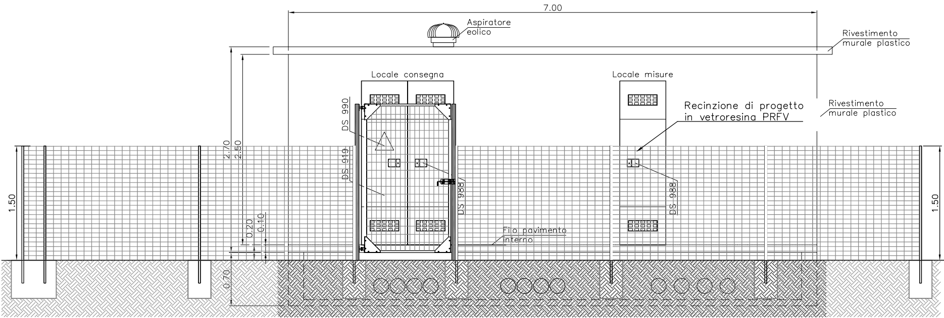
PROSPETTO FRONTALE
