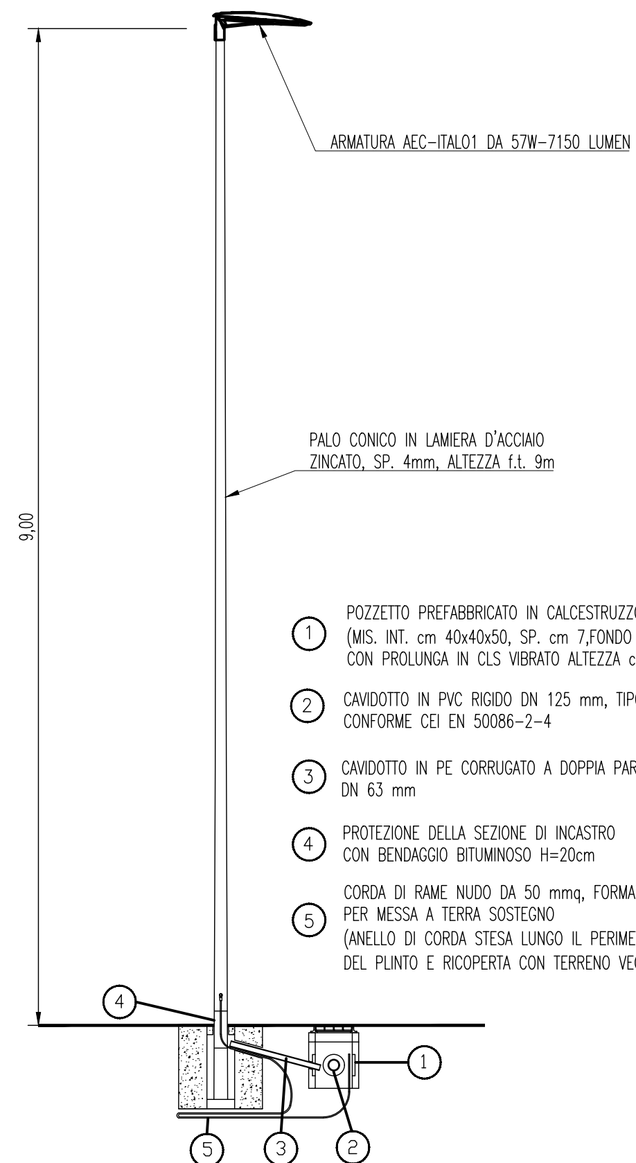
TIPICO PALO CON ATTACCO TESTAPALO (STRADA PRINCIPALI)
