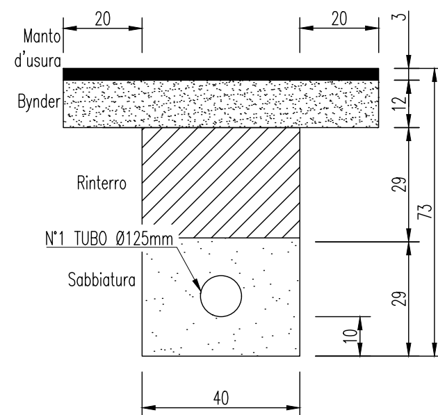
PARTICOLARE SEZIONE DI SCAVO IN TRATTO ASFALTATO (I.P.)
