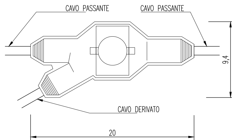
DETTAGLIO GIUNTO PER DERIVAZIONE CAVI ELETTRICI UNIPOLARI
