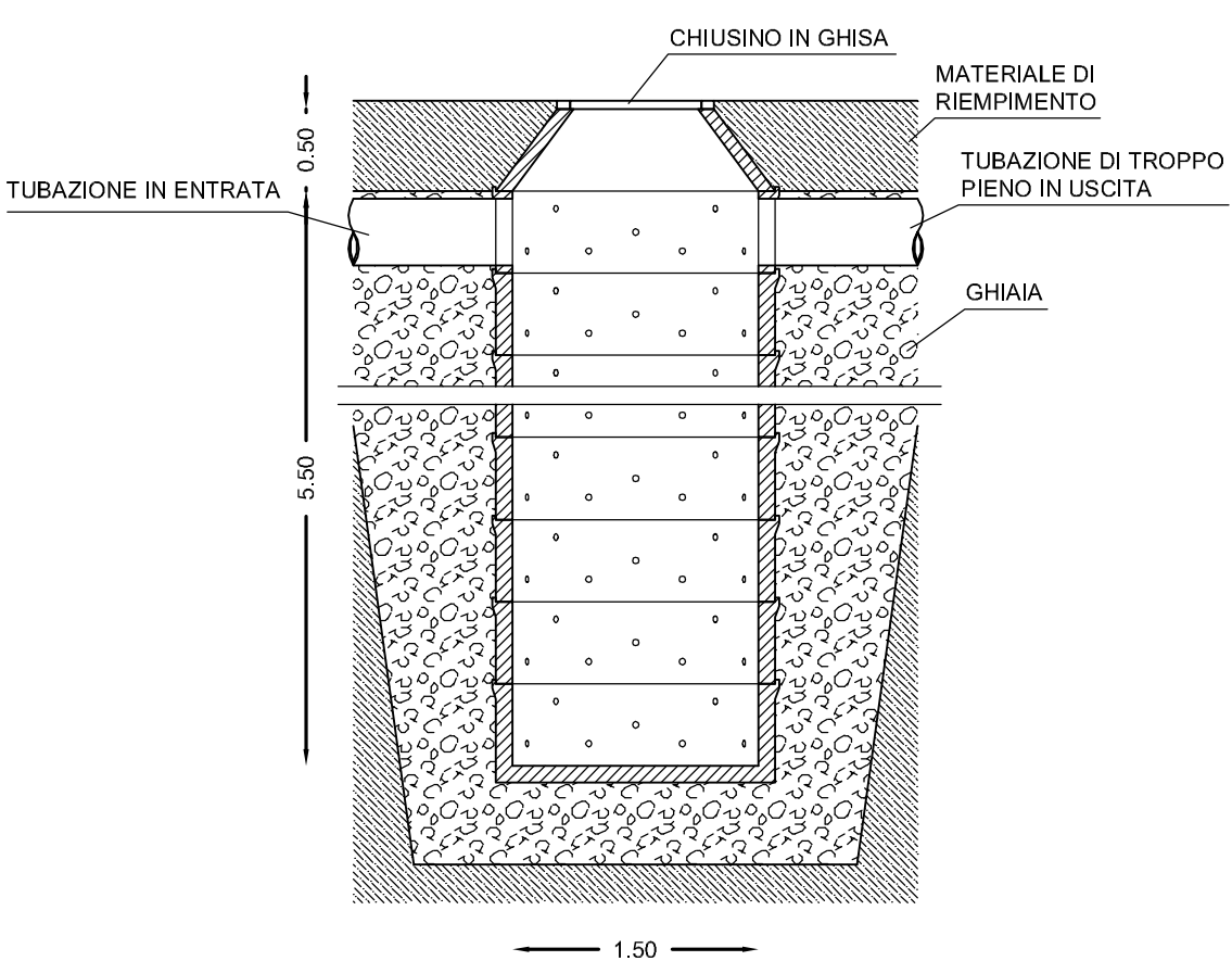
SEZIONE TIPO POZZO PERDENTE SCALA 1:50
