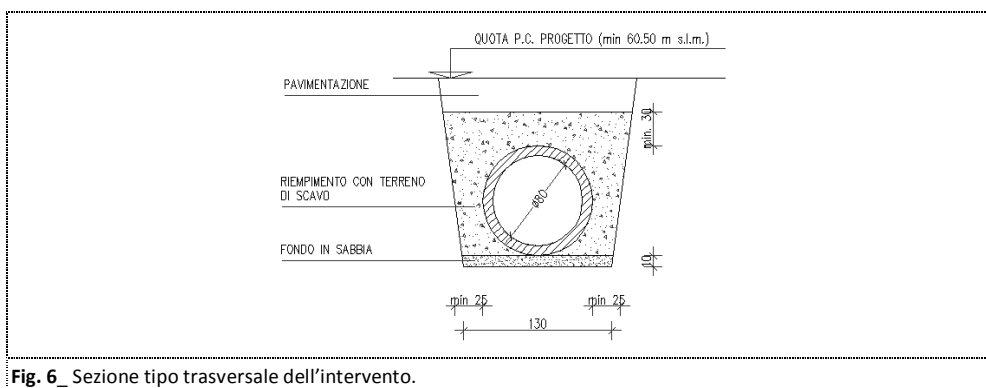
Fig. 6_ Sezione tipo trasversale dell'intervento.
