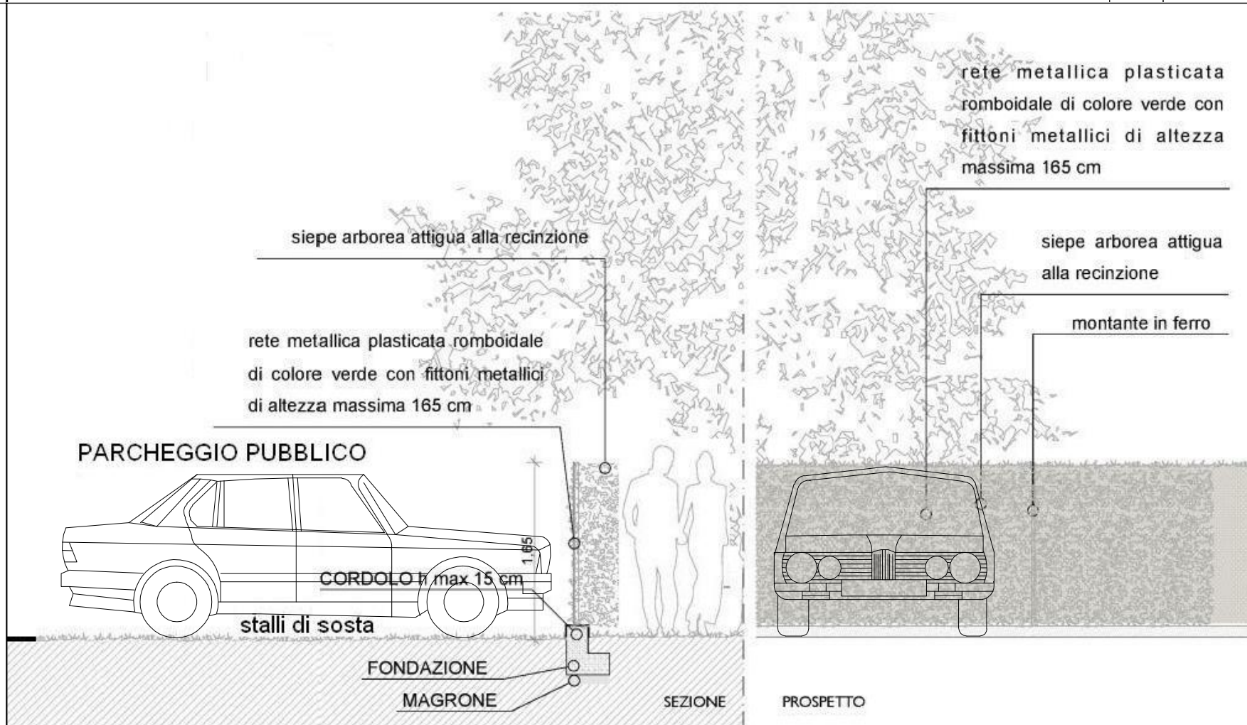
DETAGLIO RECINZIONE SCALA 1:50
