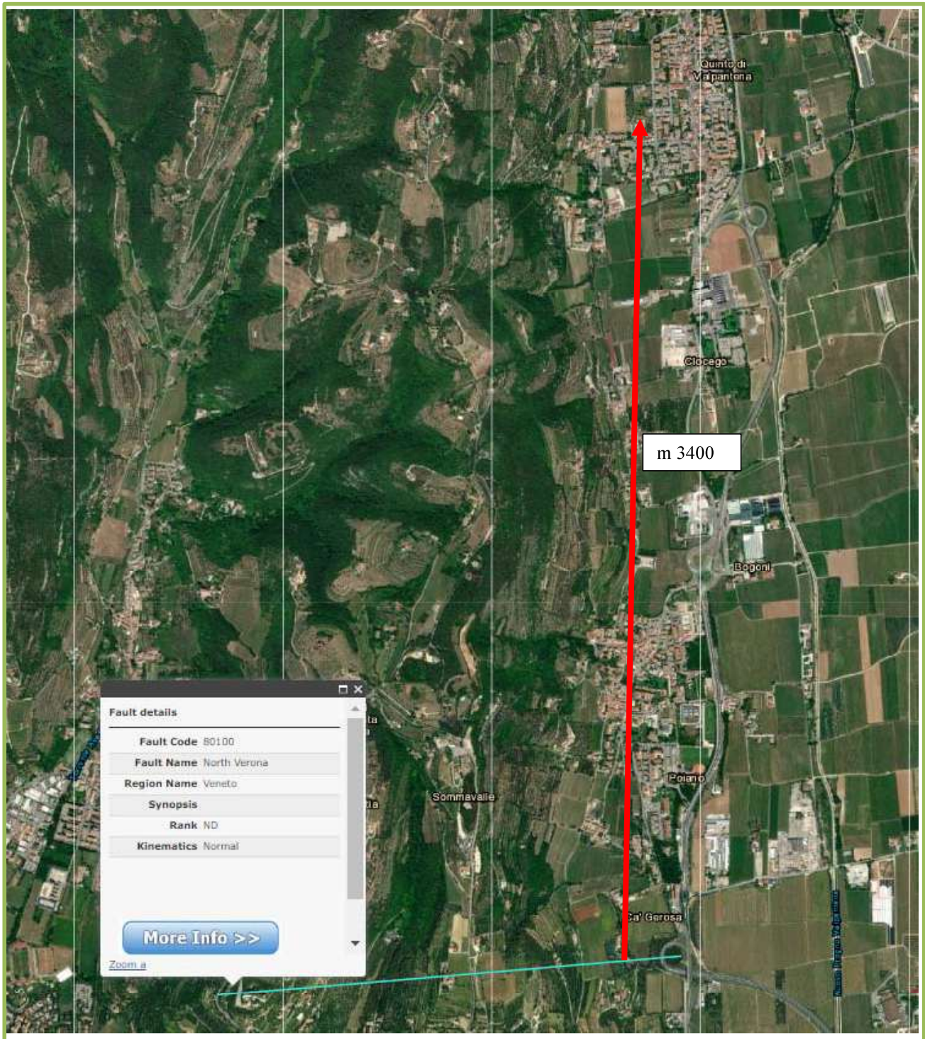
Fig. 11: posizione della faglia potenzialmente attiva e capace più vicina (progetto ITHACA)
