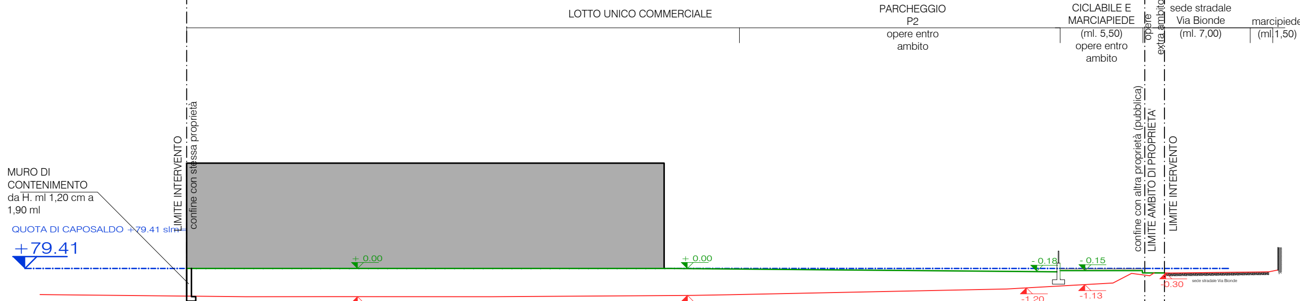
SEZIONE BB' 1:250
