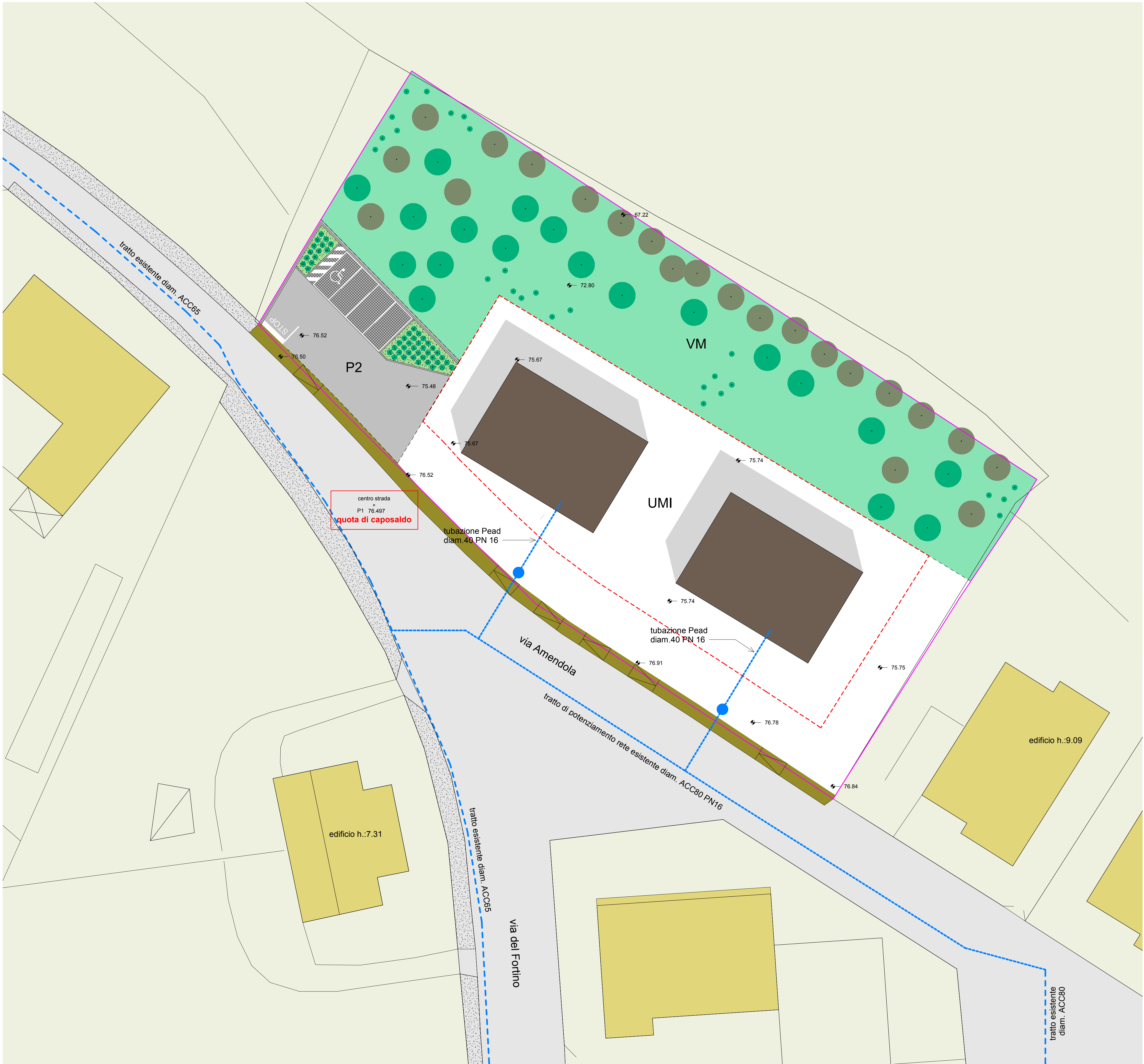
Planimetria scala 1:200
