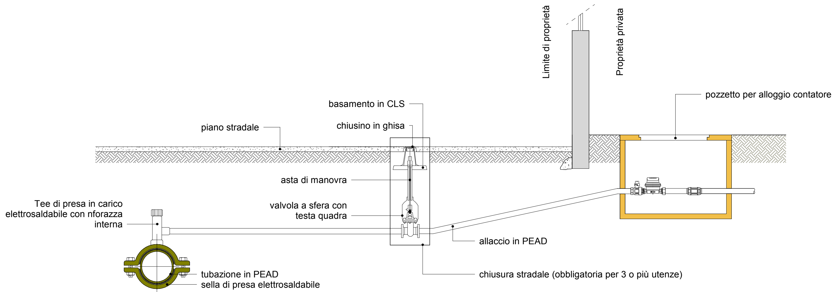
Dettaglio allaccio rete idrica
