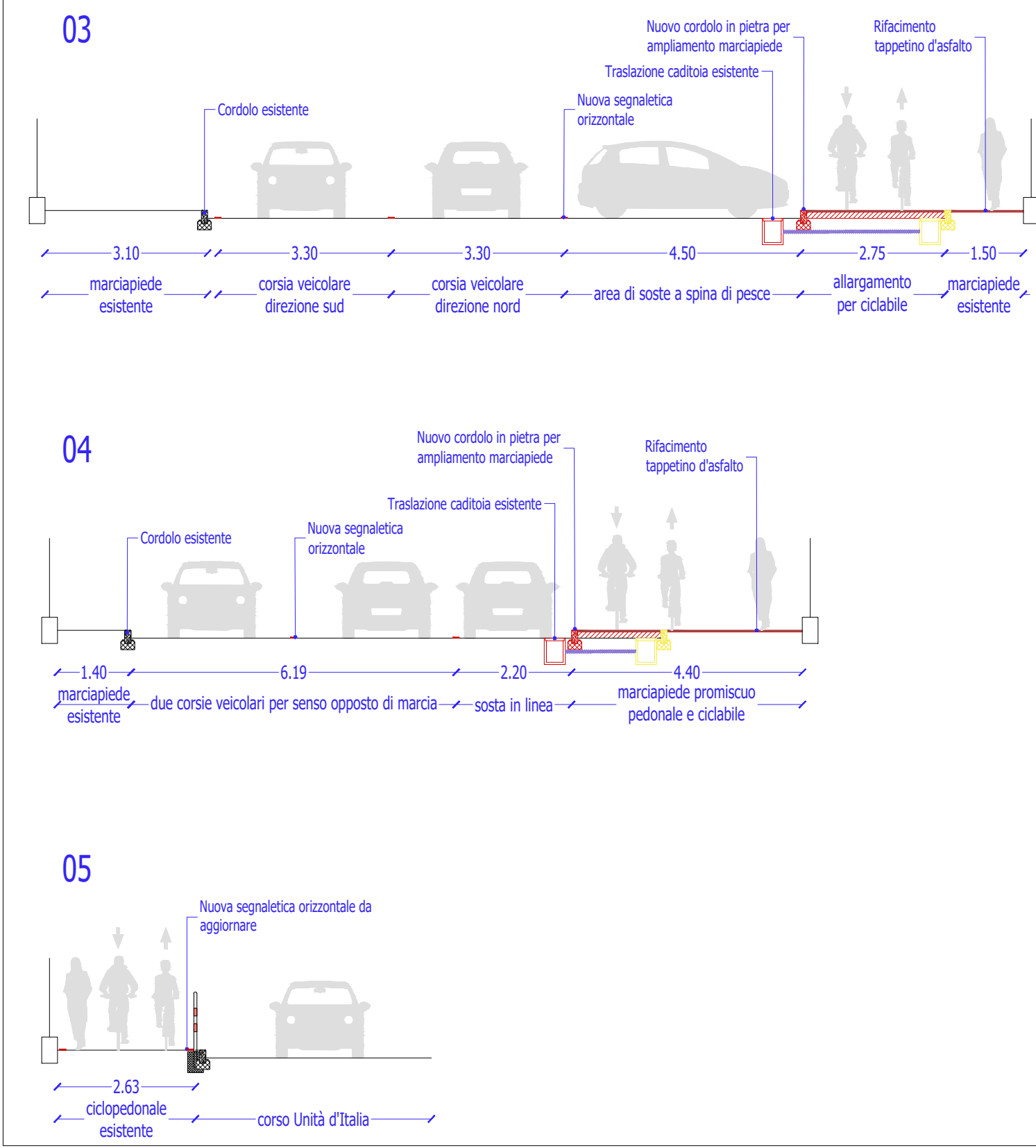
Sezioni progetto - via G. Belluzzo - Scala 1:100
