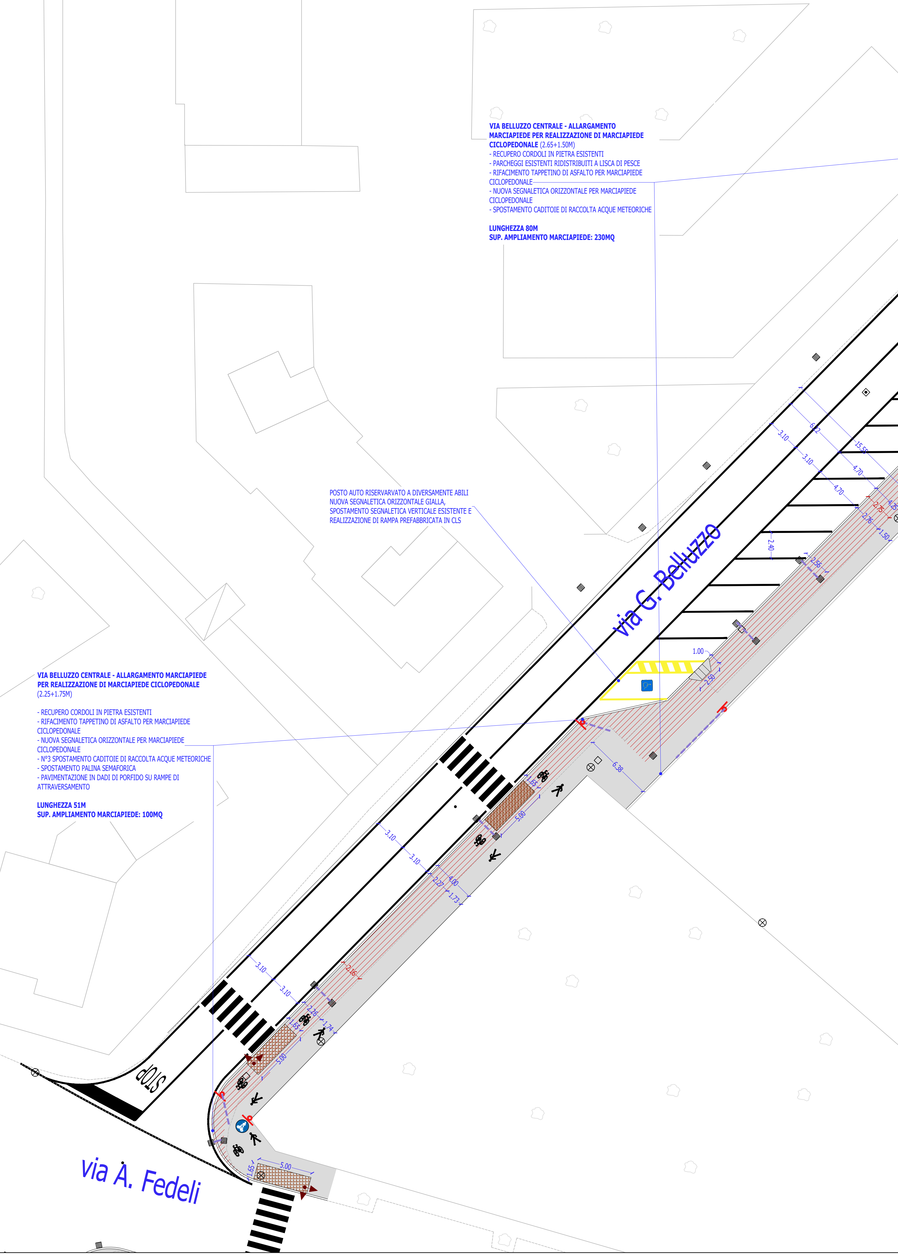
TRATTO B11 - T05 - Via G. Belluzzo tratto Centrale - Planimetria di Progetto - Scala 1:200
