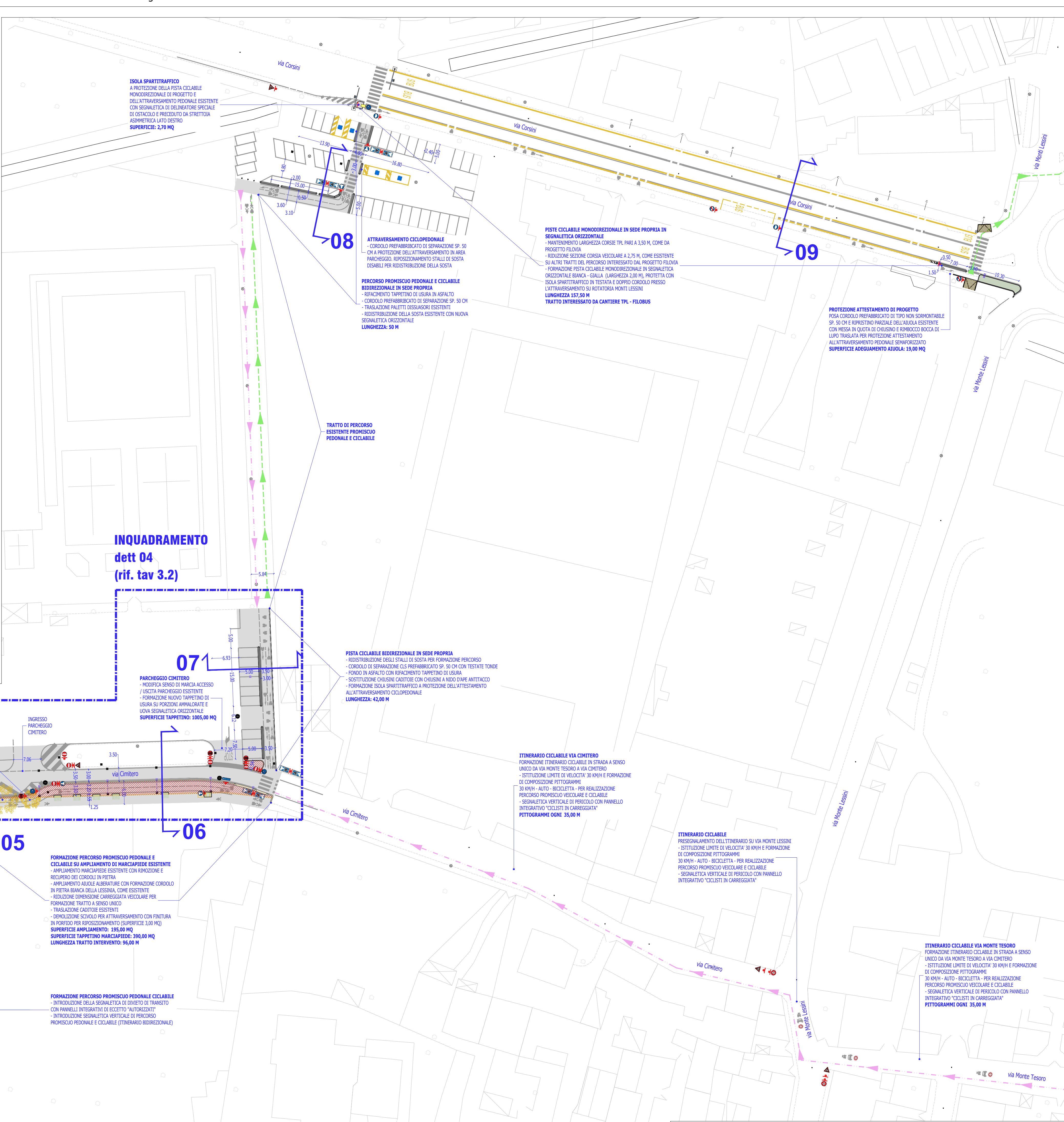
TRATTO B11 - T01 - da via Unità d'Italia a via Corsini - Planimetria di Progetto - Scala 1:500
