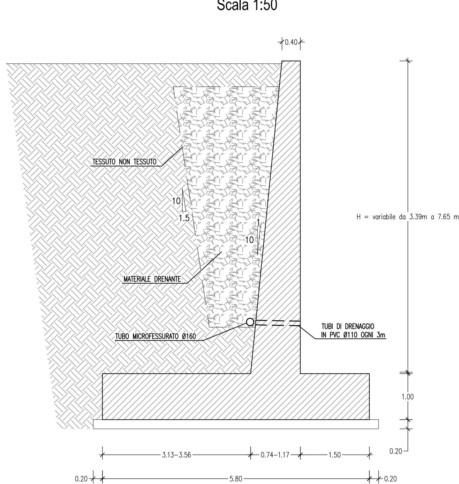
MURO TIPO Hmax=7.65
