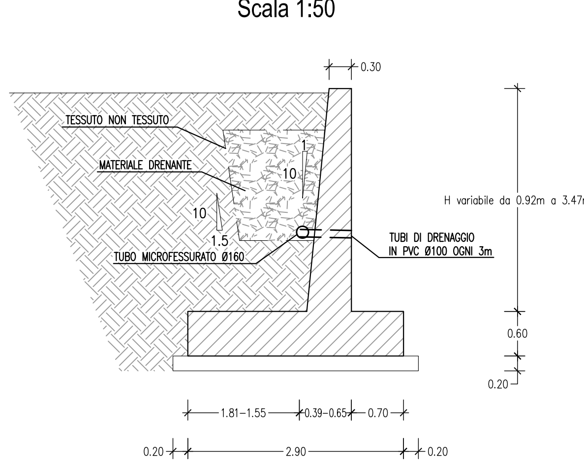
MURO TIPO Hmax=3.50
