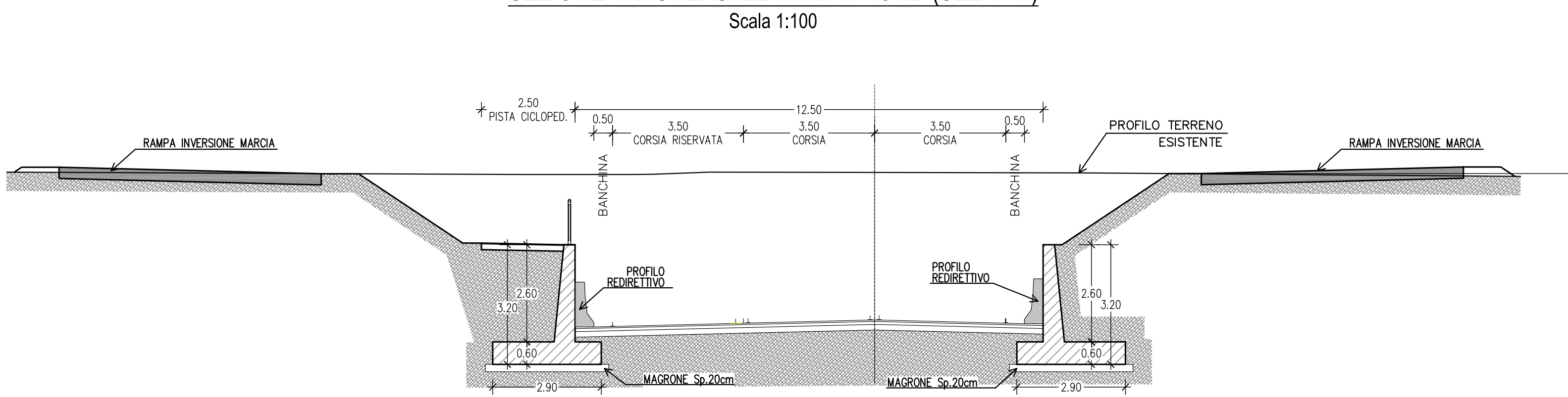
SEZIONE TRASVERSALE RAMPA NORD (SEZ. A-A)
