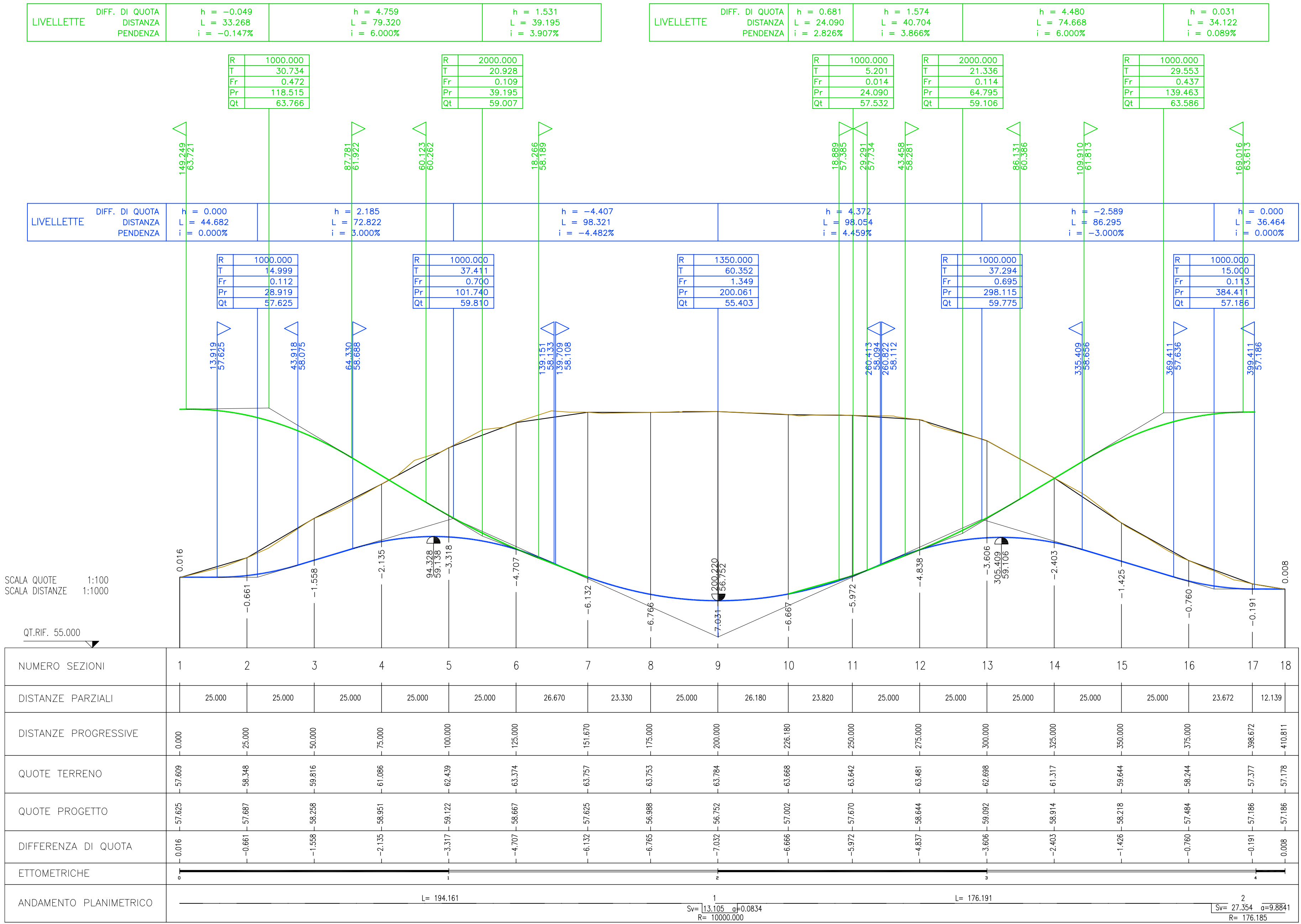
PROFILO SCALA 1:100/1:1000
