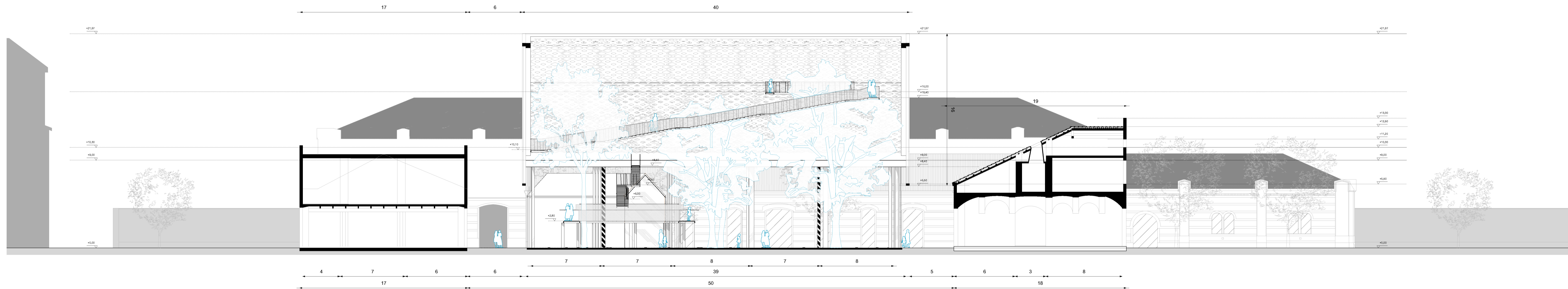
sezione trasversale A-A scala 1:200
